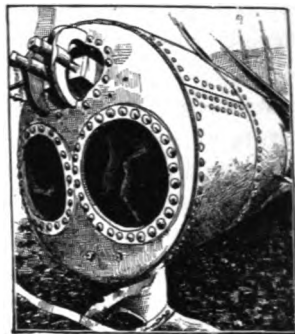
FIG. 179.—COLLAPSED FLUES.
